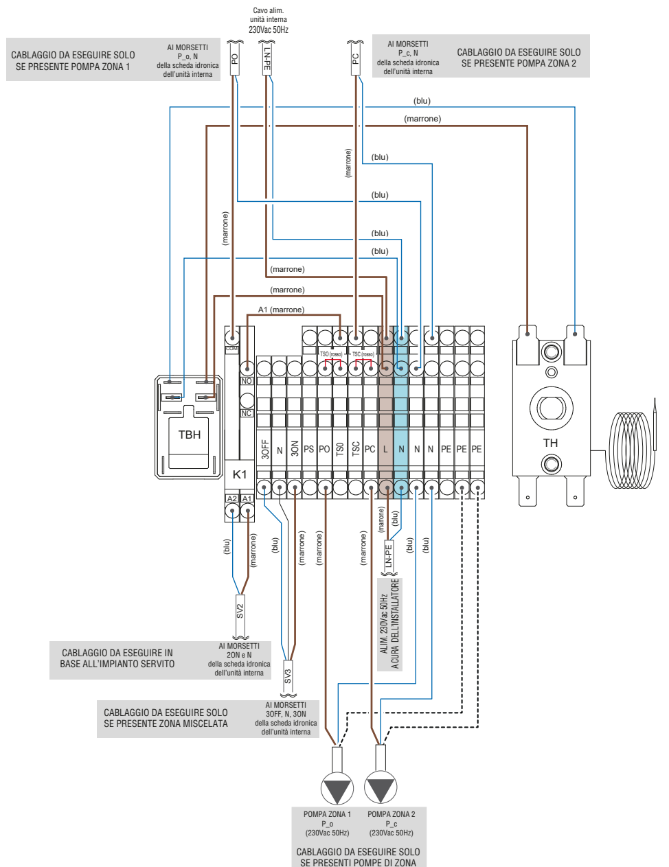
Morsettiera scheda idronica dell'unità interna
